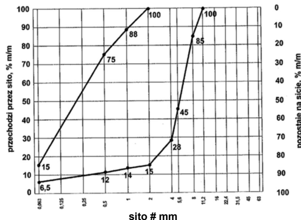
Rys. 1. Uziarnienie mieszanki CBGM 0/8
