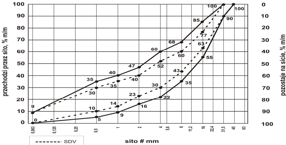
Rys.3. Uziarnienie mieszanki kruszywa przeznaczonej na warstwę podbudowy zasadniczej 0/31,5 mm
