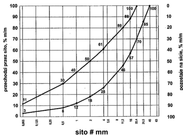
Rys. 2. Uziarnienie mieszanki CBGM 0/31,5
