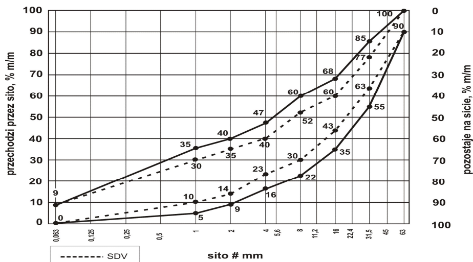
Rys.4. Uziarnienie mieszanki kruszywa przeznaczony na warstwę podbudowy zasadniczej 0/63 mm
